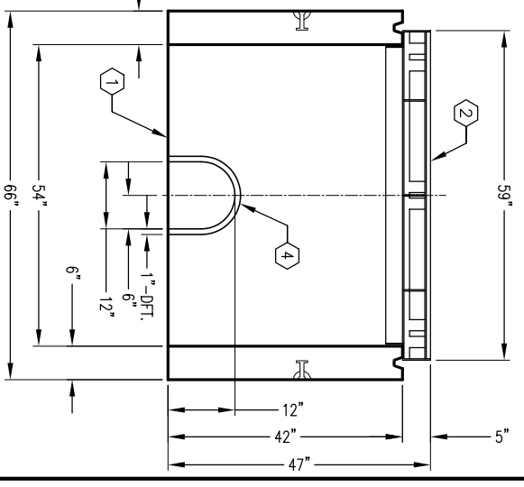
SECTION D-D
